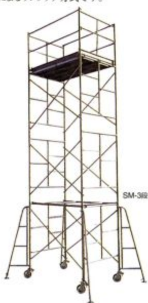
■ハセガワ ローリングタワー SM型の仕様 最大使用重量: 200kg
