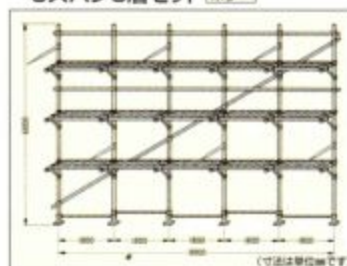
■ホリー 一側足場(ブラケットタイプ)5スパン3層セットの仕様
